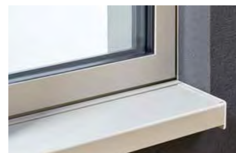
Designfensterbank ALU, DS2 – keine sichtbare Verschraubung zum Fensterrahmen hin.
